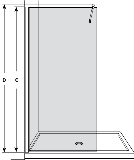
Shower shield with suport bar an angle Écran de douche avec barre de support en angle
