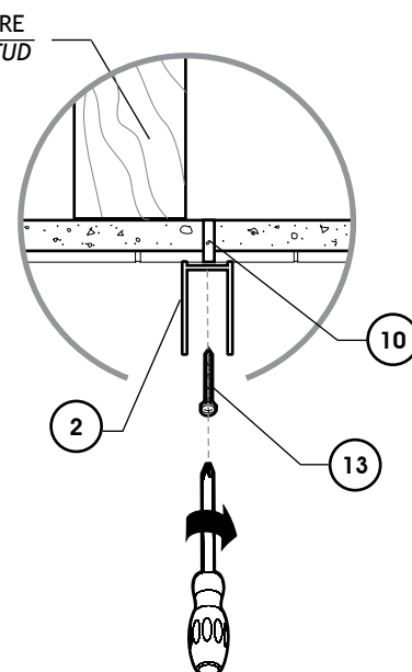
1C(b) VUE DU HAUT TOP VIEW
